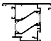
PR65126 Kontra krilo vrata
