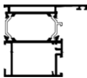
PR65106 Štok širi
