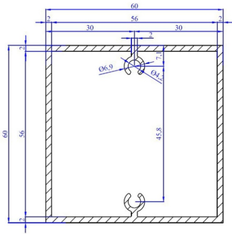
ÖLÇEK / SCALE 1 / 2
