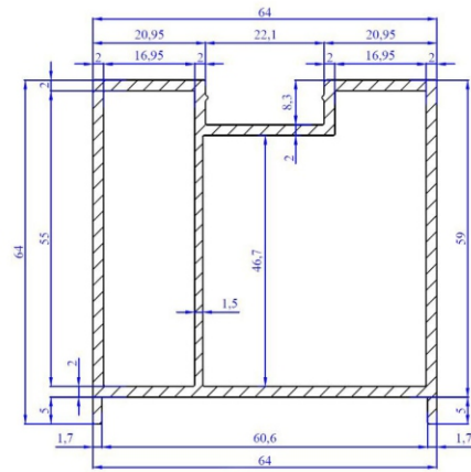
ÖLÇEK / SCALE 1 / 2
